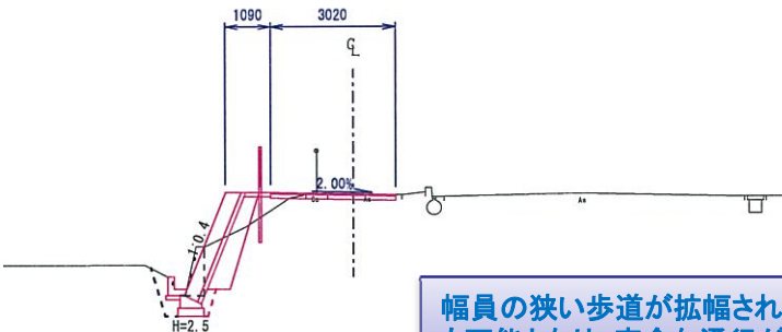
標準横断面図
