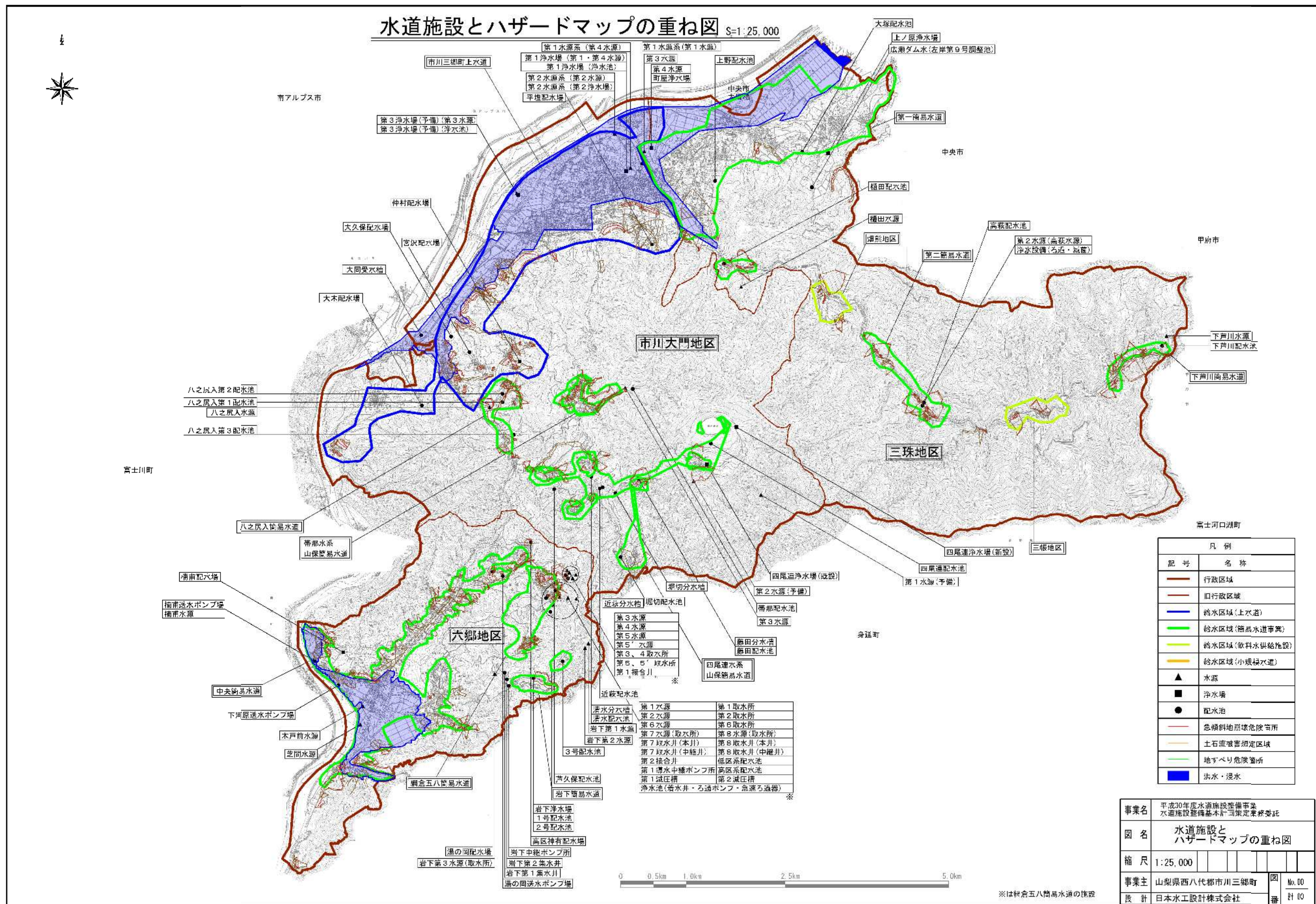
図2-3-2 市川三郷町の水道施設とハザードマップの重ね図
